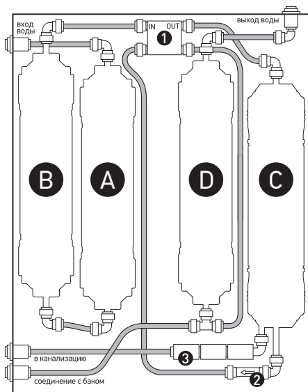
Рис. 2. Схема основного блока системы Expert Osmos M0510/M0520.
